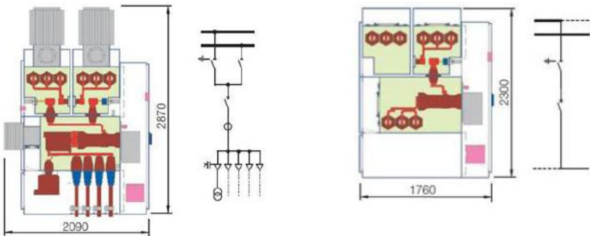
图B. 5a 型式试验过的功能单元（无散热器版）图B. 5b 母联功能单元
