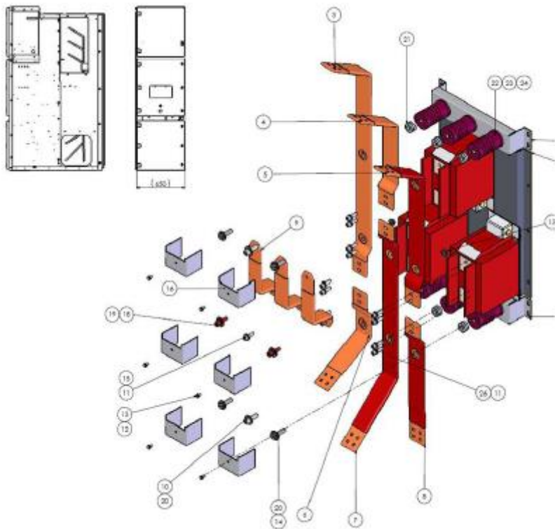
图B. 2 空气绝缘开关设备的立柱母线功能单元中增加的块式电流互感器
