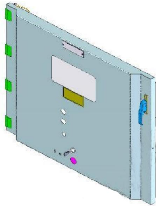
图B. 3 用特殊类型钥匙锁代替空气绝缘开关设备门上的标准钥匙锁
